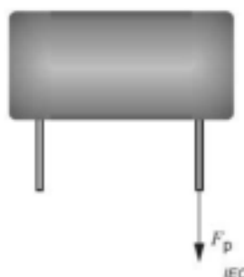
b) Force de traction F_p appliquée sur un spécimen avec sorties par fils radiales
