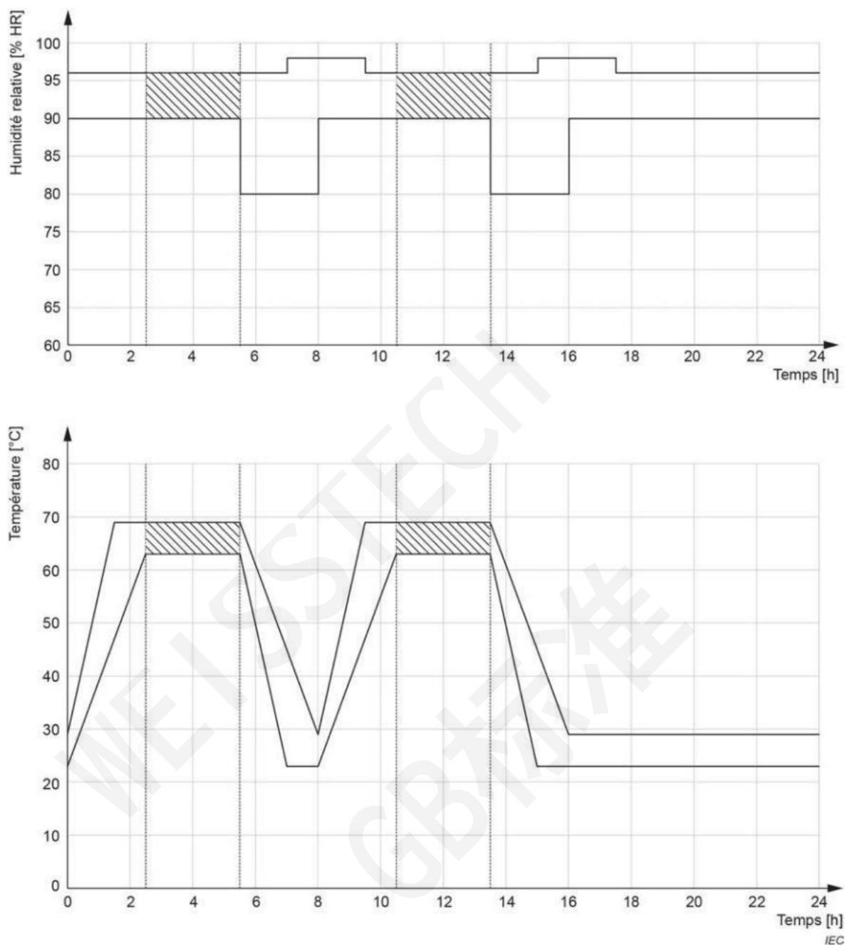
Figure 5 – Durées d'essai pour le fonctionnement intermittent du spécimen – Exposition à l'humidité, non suivie d'une exposition au froid
