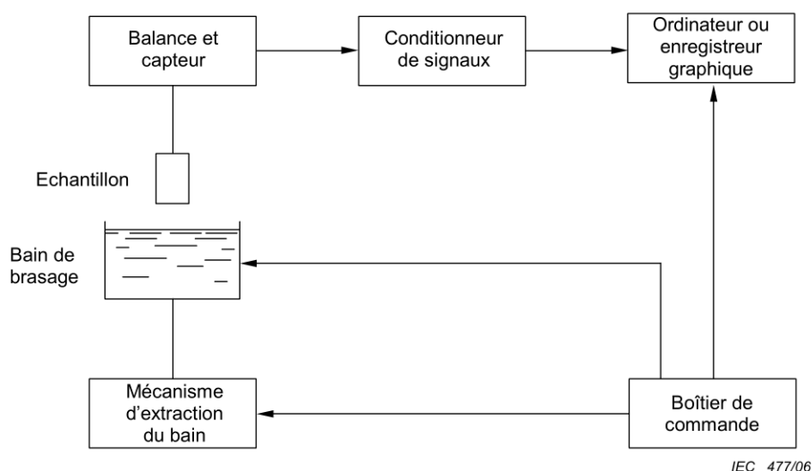
Figure 1 – Organisation d'essai
