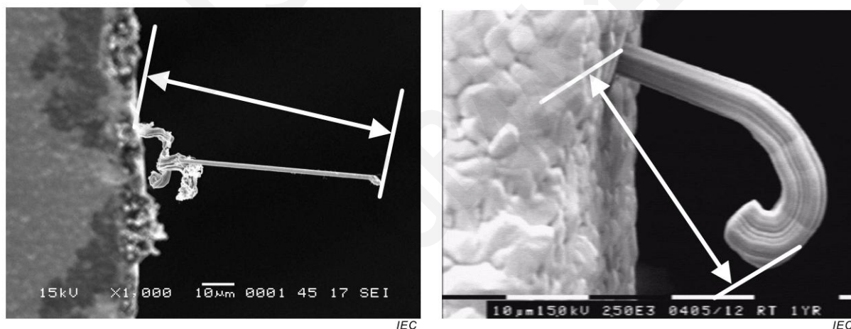
Figure A.2 – Exemple du mesurage de la longueur des trichites
