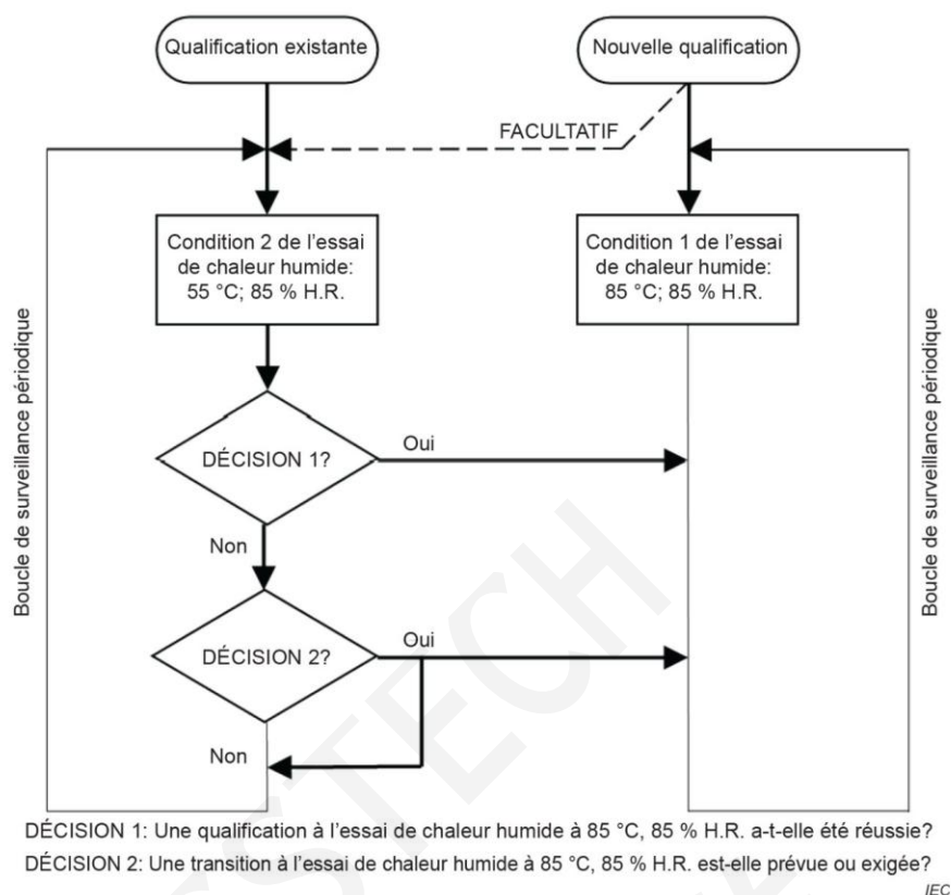
Figure E.1 – Voies de transition pour les essais de chaleur humide de composants
