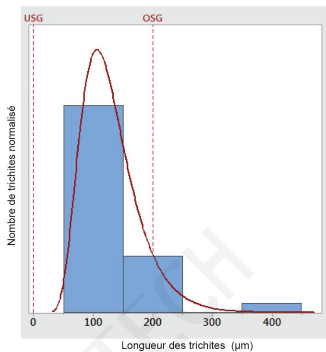
Figure C.4 – Histogramme des longueurs des trichites et distribution log-normale ajustée
