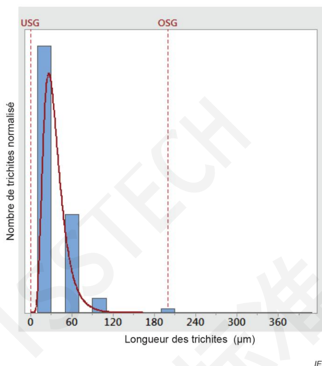
Figure C.3 – Histogramme des longueurs des trichites et distribution log-normale ajustée
