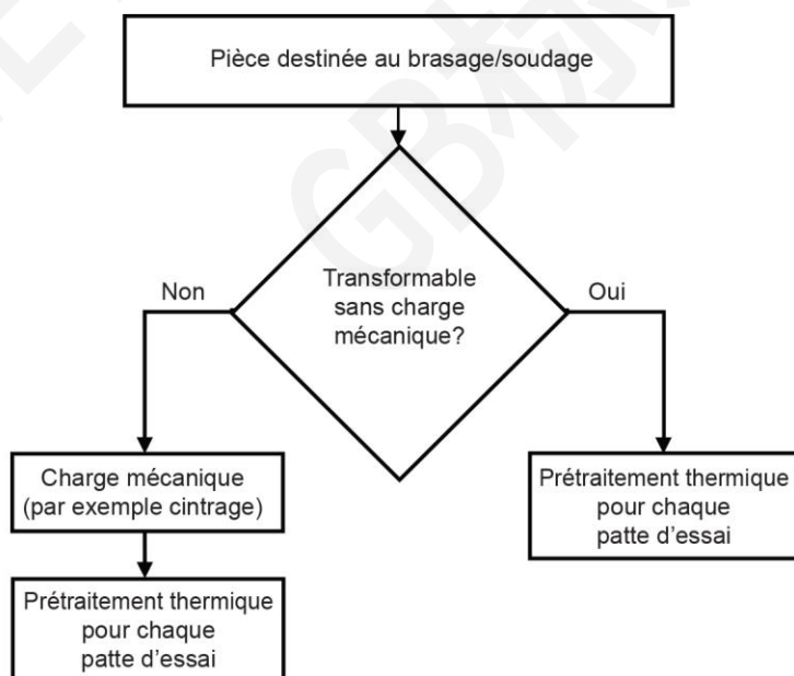
Figure 3 – Flux de traitement et/ou cintrage et traitement thermique
