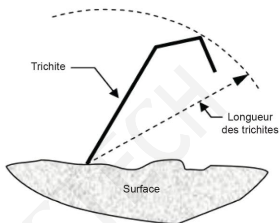
Figure A.1 – Estimation de la longueur des trichites
