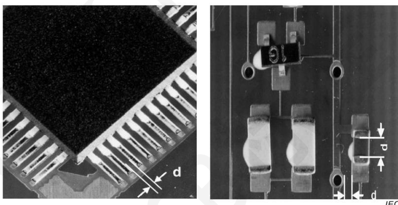
Figure C.1 – Plus petite distance des composants et des cartes de circuits imprimés
