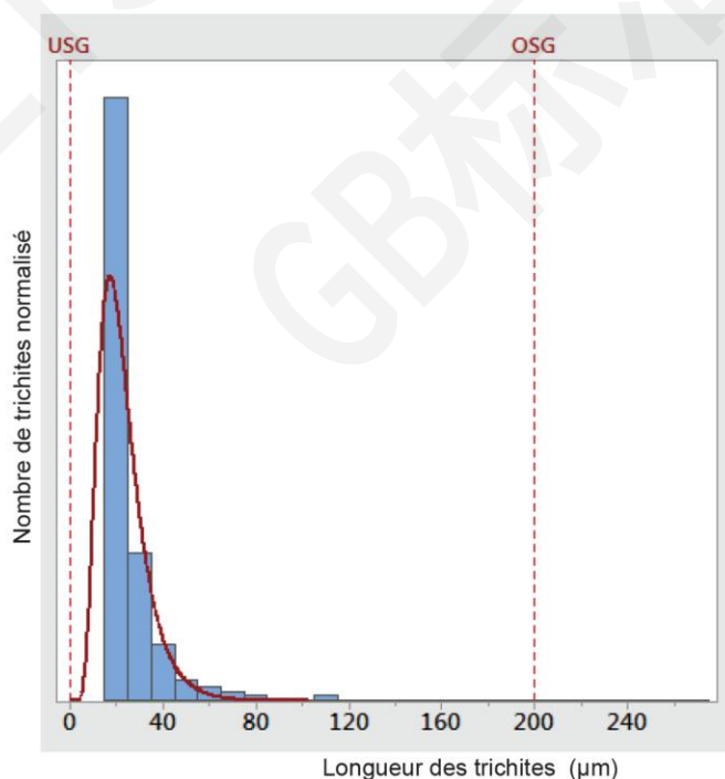
Figure C.2 – Histogramme des longueurs des trichites et distribution log-normale ajustée
