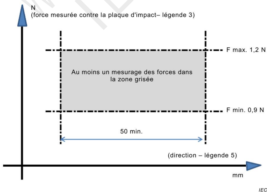
Figure D.9 – Répartition de la force d'impact
