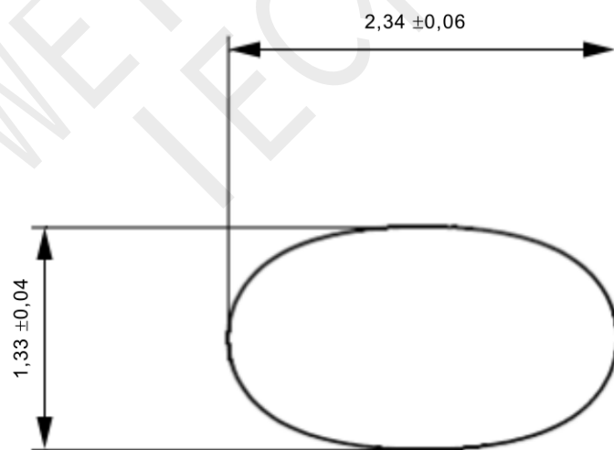
Figure D.6 – Dimensions du trou d'arrosage obtenu avec la buse à jet en éventail à des fins de vérification
