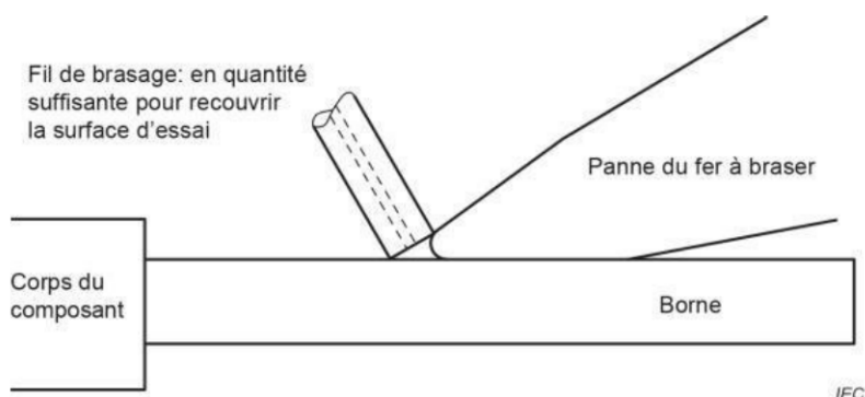
Figure 2 – Position du fer à braser
