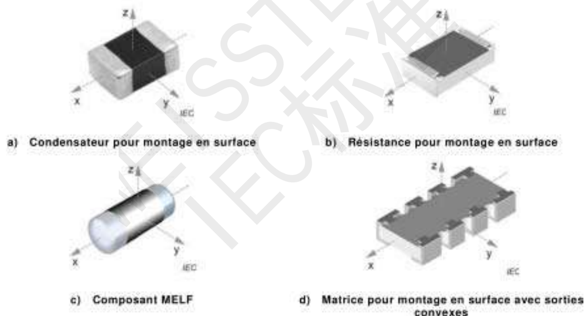
Figure 23 – Exemples d'application de l'essai Uf_2 de choc par impact sur le corps d'un CMS
