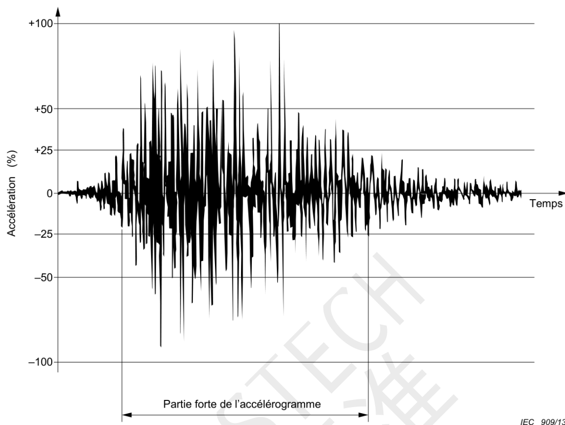
Figure 3 – Accélérogramme caractéristique
