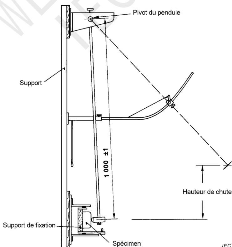
Figure D.1 – Appareillage d'essai
