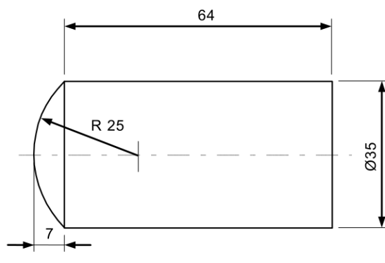
Figure A.2 – Exemple de pièce de frappe pour une valeur 2 J
