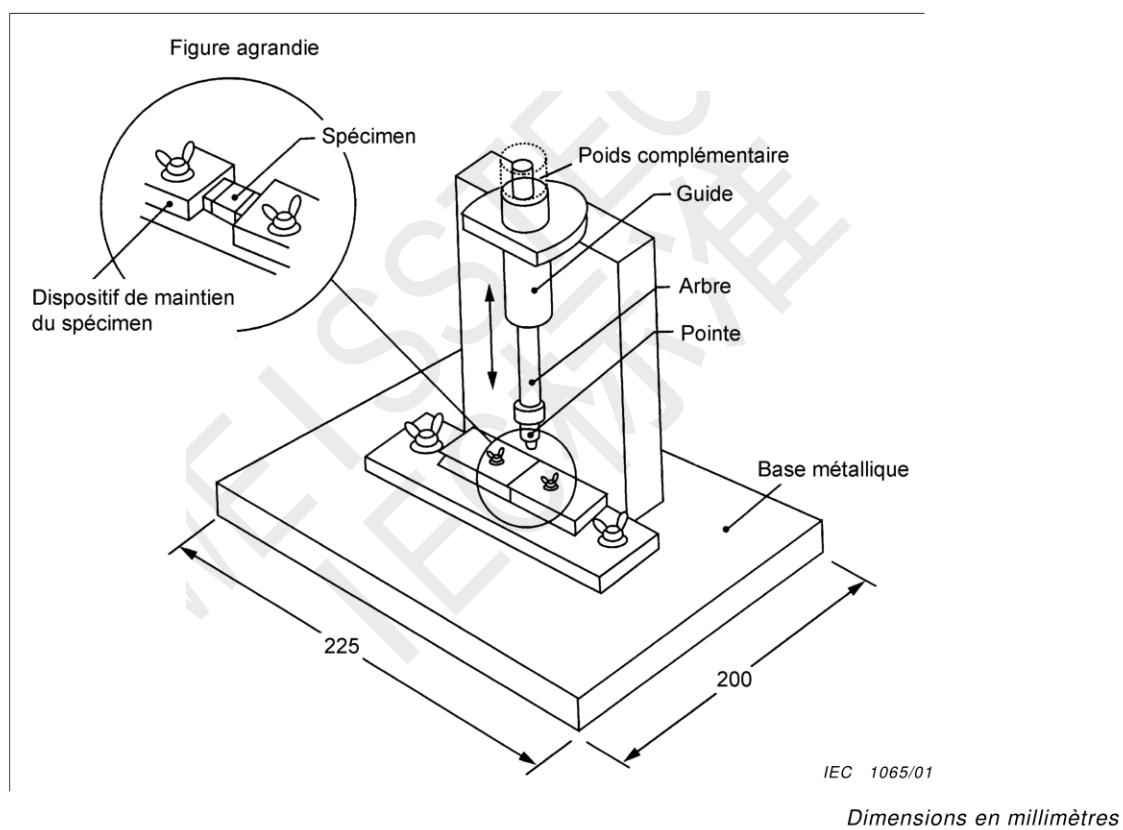
Figure 5 – Exemple d'équipement d'essai de chocs par impact
