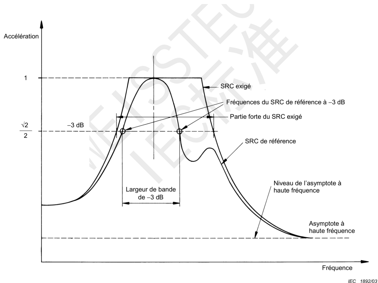
Figure B.1 – Partie forte du SRS
