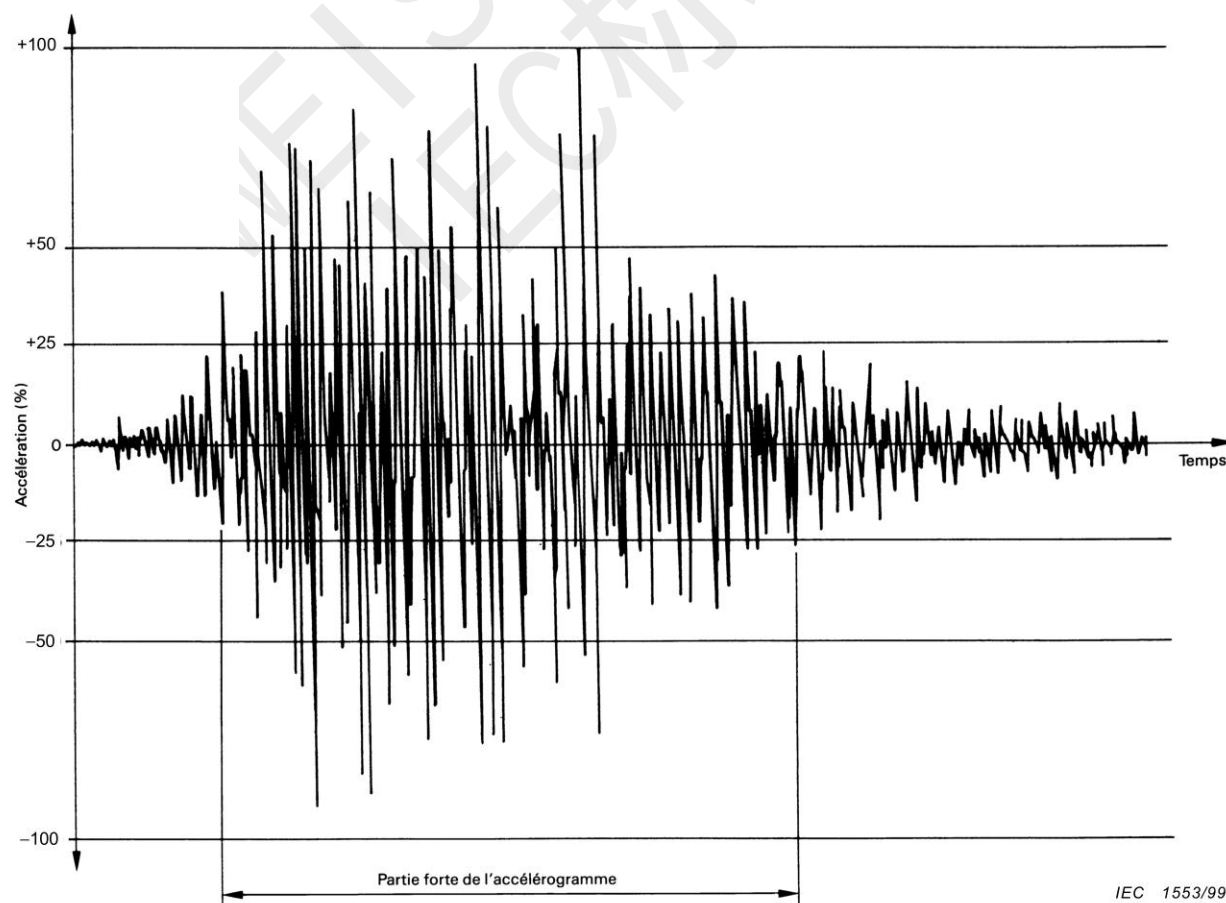
Figure 4 – Accélérogramme typique
