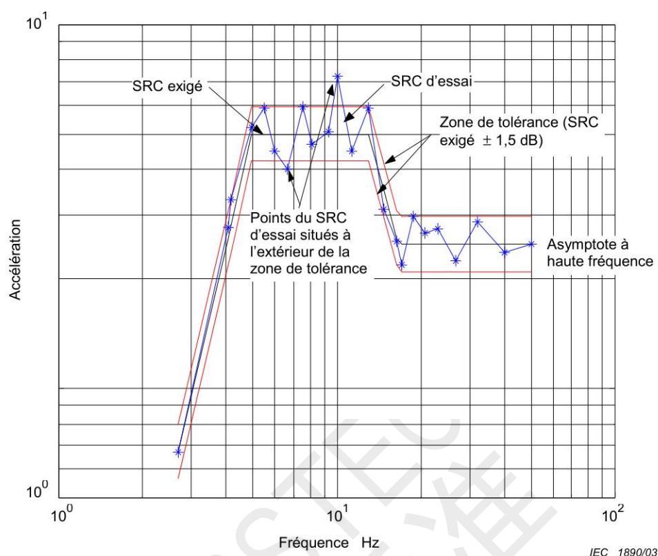
Figure 3 – Graphique logarithmique typique d'un SRC exigé
