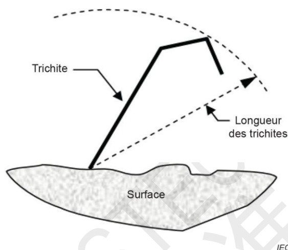
Figure A.1 – Estimation de la longueur des trichites
