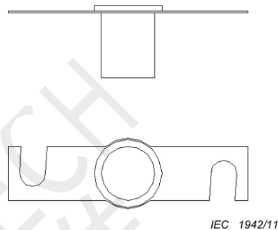
Figure 7b – Mini creuset
