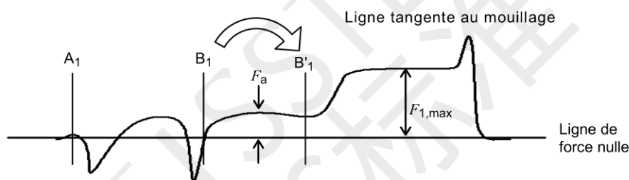
Figure B.3 – Exemple de correction de l'instant initial de mouillage ( F_a est inférieure ou égale à 0,5F_{1,max} )
